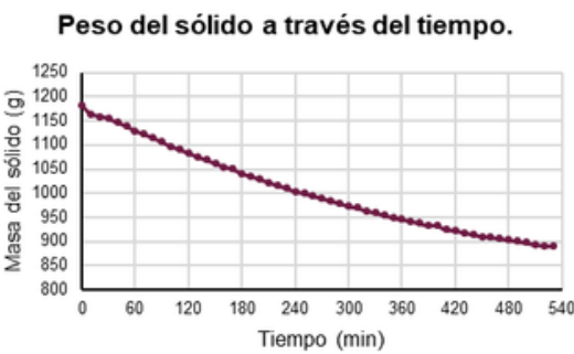
Figura 2. Comportamiento del peso a través del tiempo de operación.
