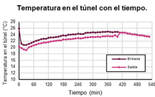
Figura 4. Comportamiento de la temperatura de entrada y salida del túnel de secado a través del tiempo de operación.
