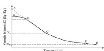
Figura 1. Cinética de la humedad en el secado.
